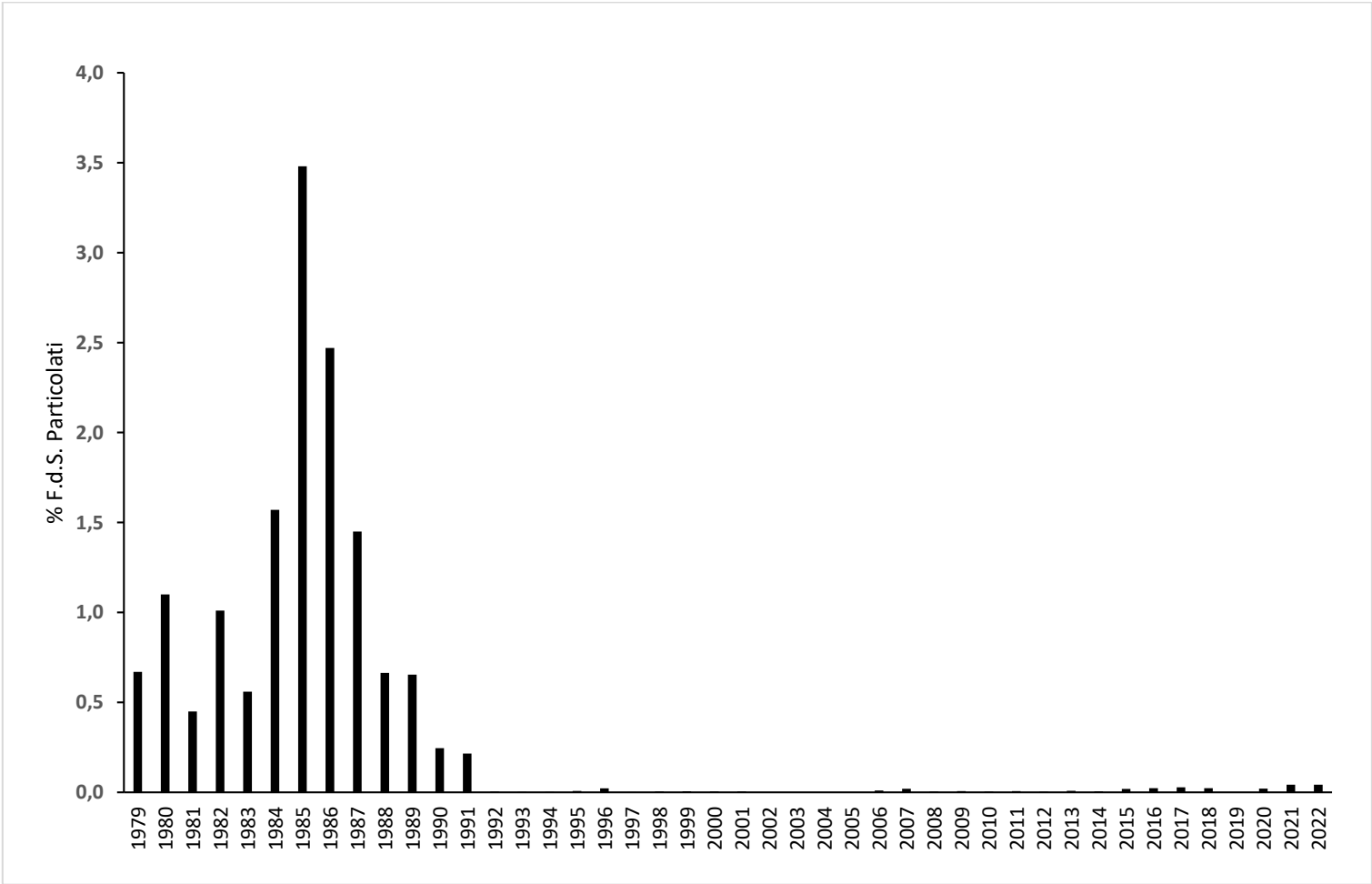
Figura 2: Andamento % Formula di Scarico Particolati
